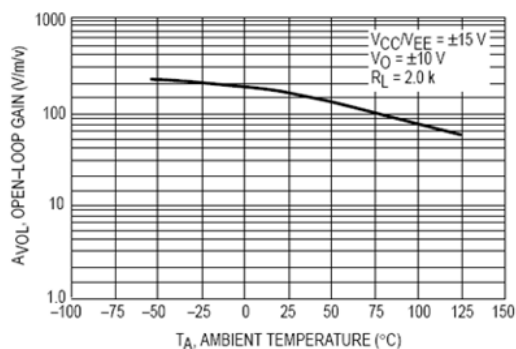
图10 大信号电压增益与温度的关系曲线
