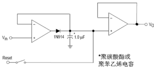
图 14 正峰值检测器
