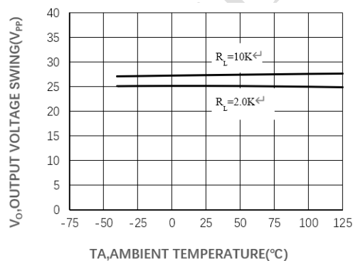
图7 输出电压摆幅与温度的关系曲线
