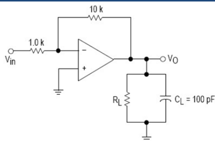
图2 反向放大器增益为 10
