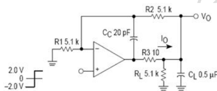
图 15 电压控制电流源
