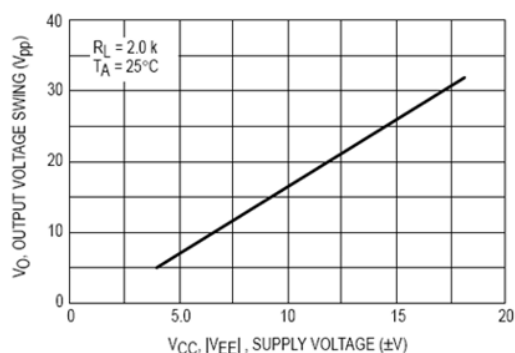
图6 输出电压摆幅与供电电压的关系曲线
