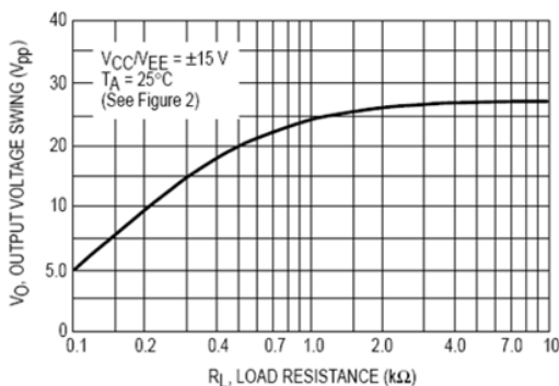
图5 输出电压摆幅与负载电阻的关系曲线
