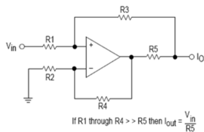
图 15 电压控制电流源
