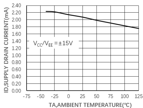
图8 每个放大器的供电电流与温度的关系曲线
