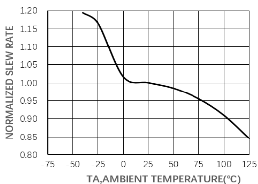
图11 标准的限摆率与温度的关系曲线
